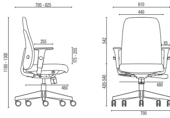
40.101 Giratoria Alta
