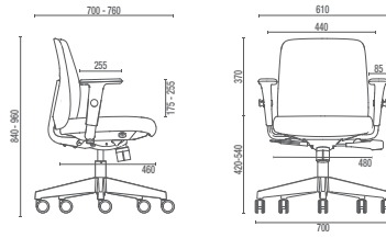
40.102 / 40.202 Giratoria Mediana
