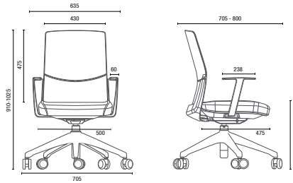
17.301 Giratoria – Brazo TC y Base Up
