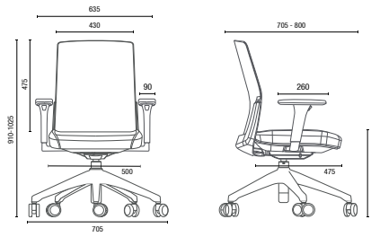
17.101 Giratoria – Brazo MC y Base Up
