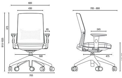
17.201 Giratoria – Brazo SL y Base Up
